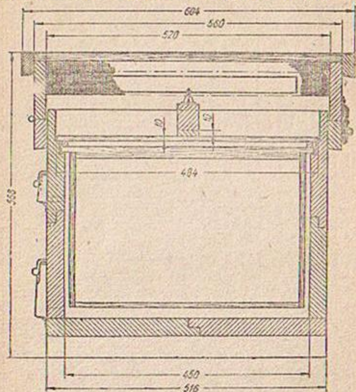
Fig. 22— Stupul orizontal (secţiune perpendiculară pe urdiniş)
