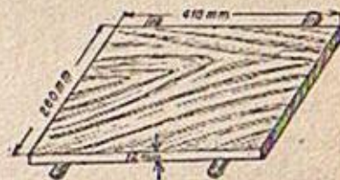
Fig. 29 — Calapodul pentru fixarea în rame a foilor de faguri artificiali
