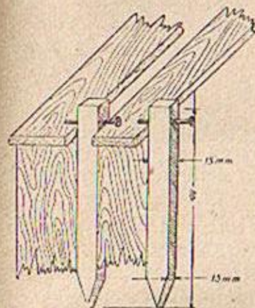
Fig. 63—Distanțătoare mobile ce se introduc între rame, pentru fixarea lor în timpul transportului
